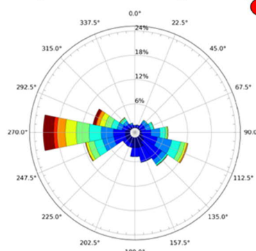
Übergeordnete Windrichtungsverteilung
